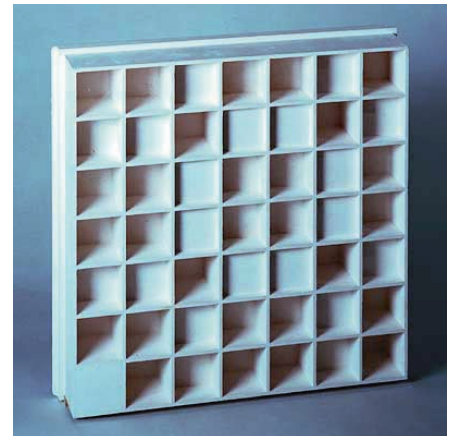
Omniffusor® FRG 2D-Diffusor aus faserverstärktem Gips, nicht brennbar
