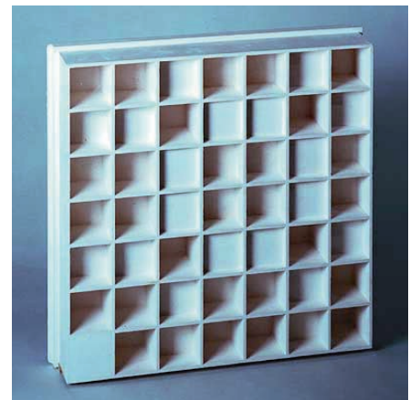
Omniffusor® FRG 2D-Diffusor aus faserverstärktem Gips, nicht brennbar
