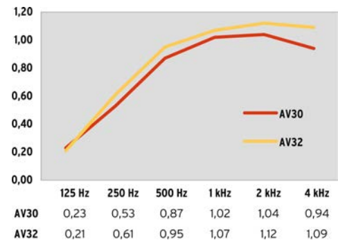
Schallabsorptionsgrad bei 1,7-fachem Faltenwurf und Wandabstand 15 cm
